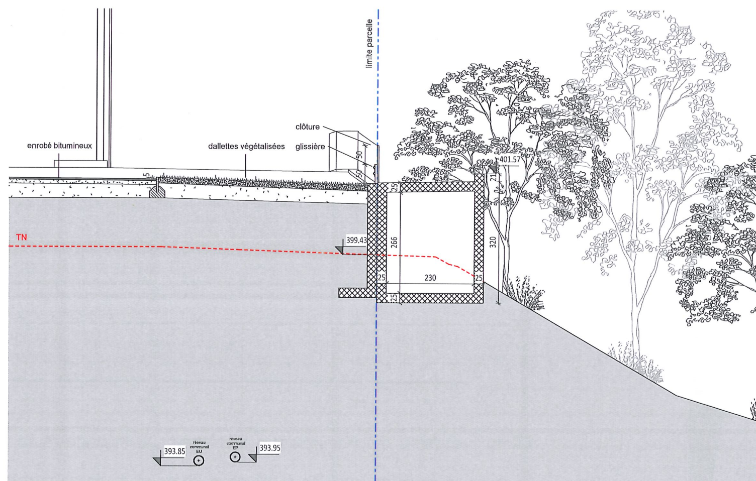
Coupe BB 1:100
