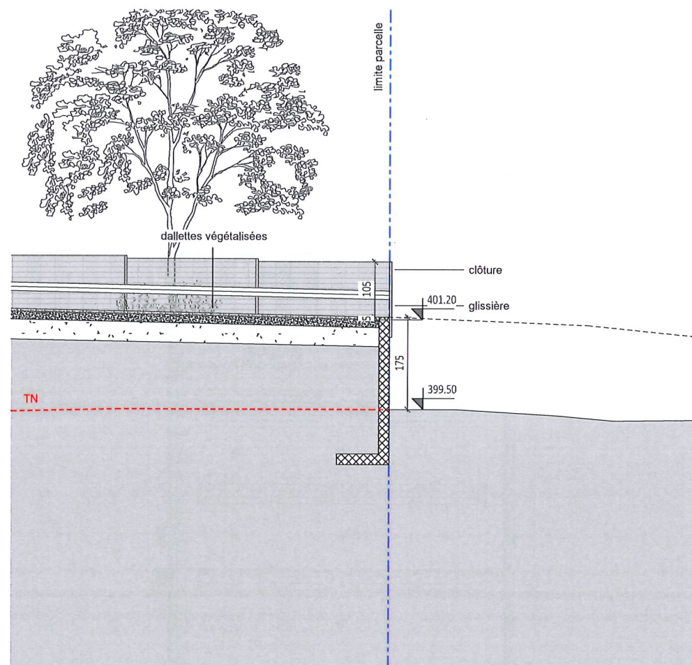
Coupe AA 1:100
