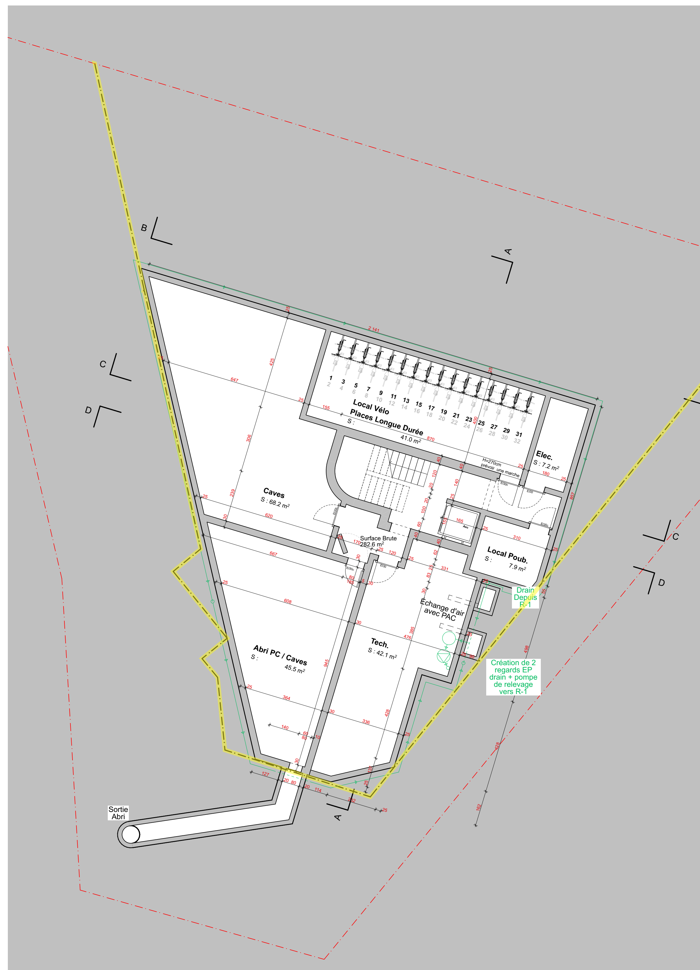
Sous-sol -2 et canalisations
