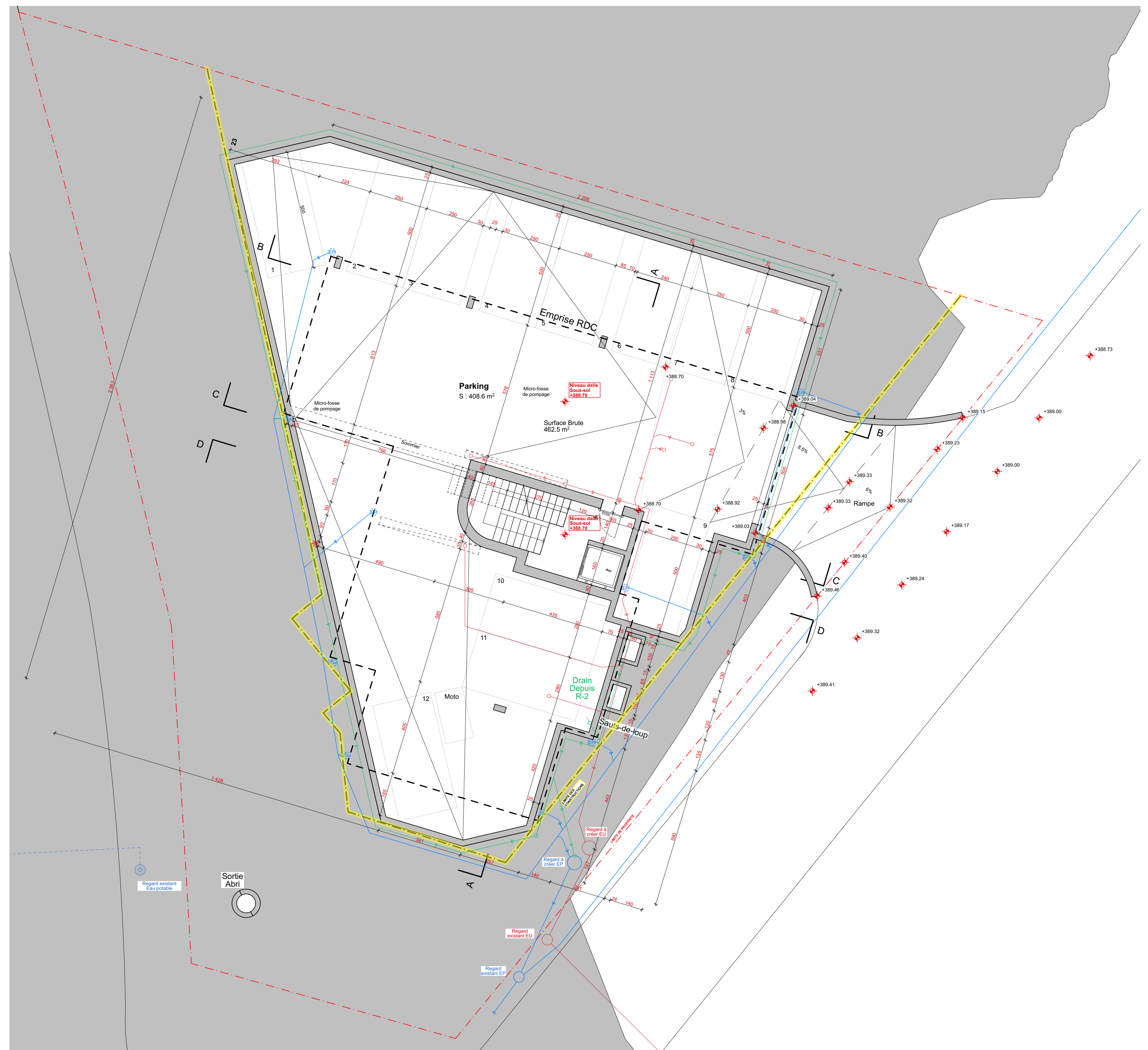
Sous-sol -1 et canalisations
