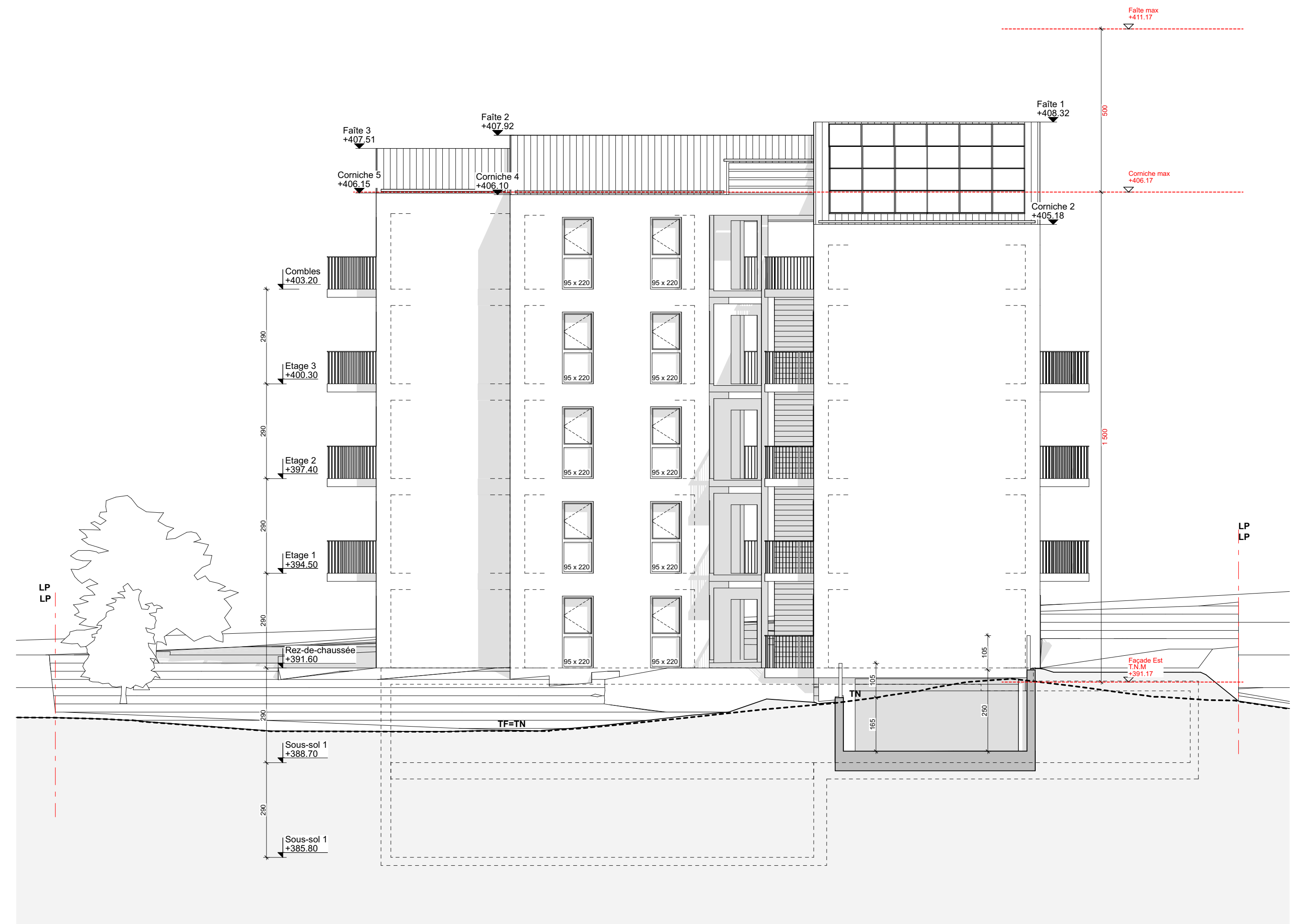
Façade Est
