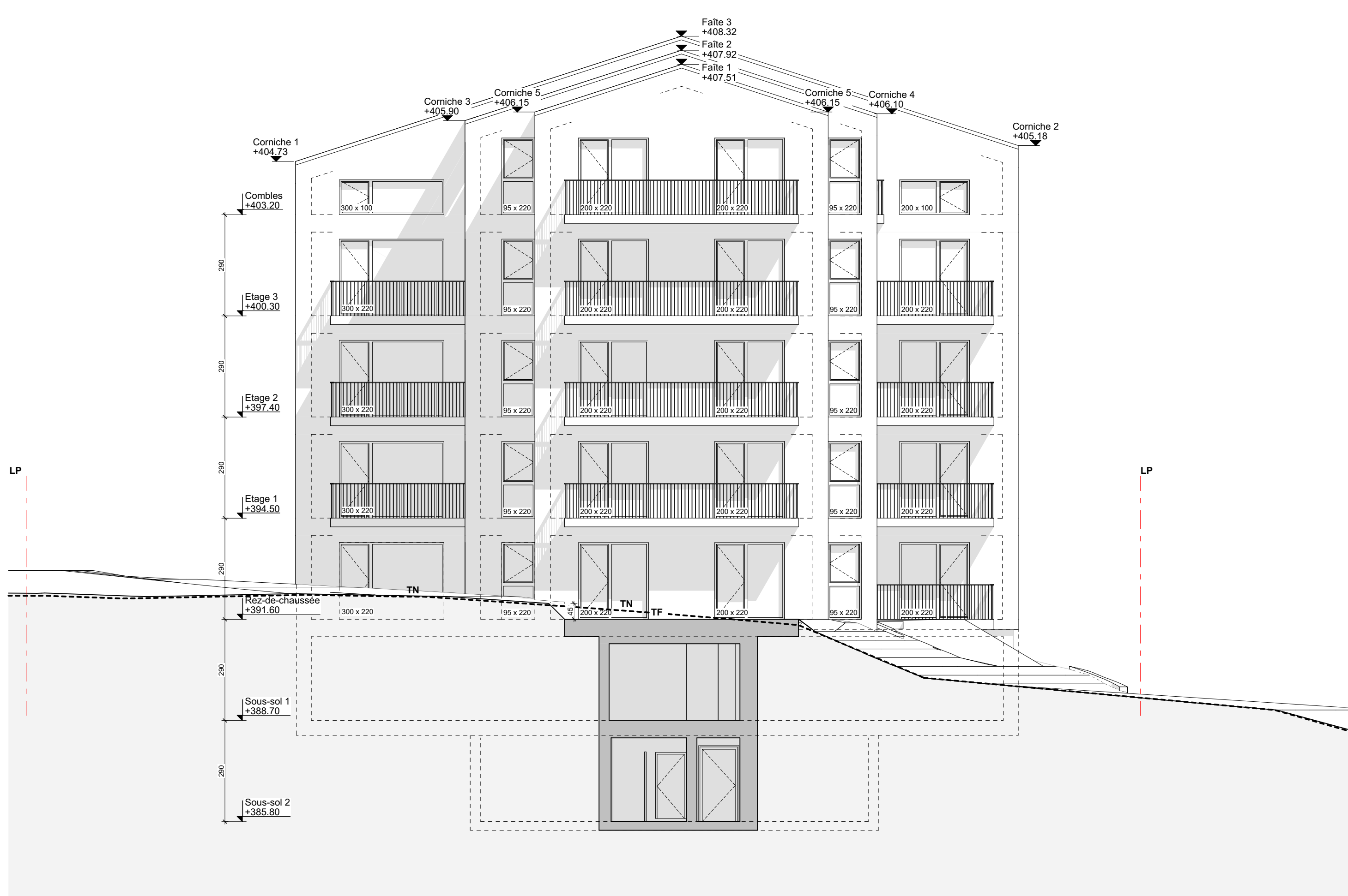
Façade Sud
