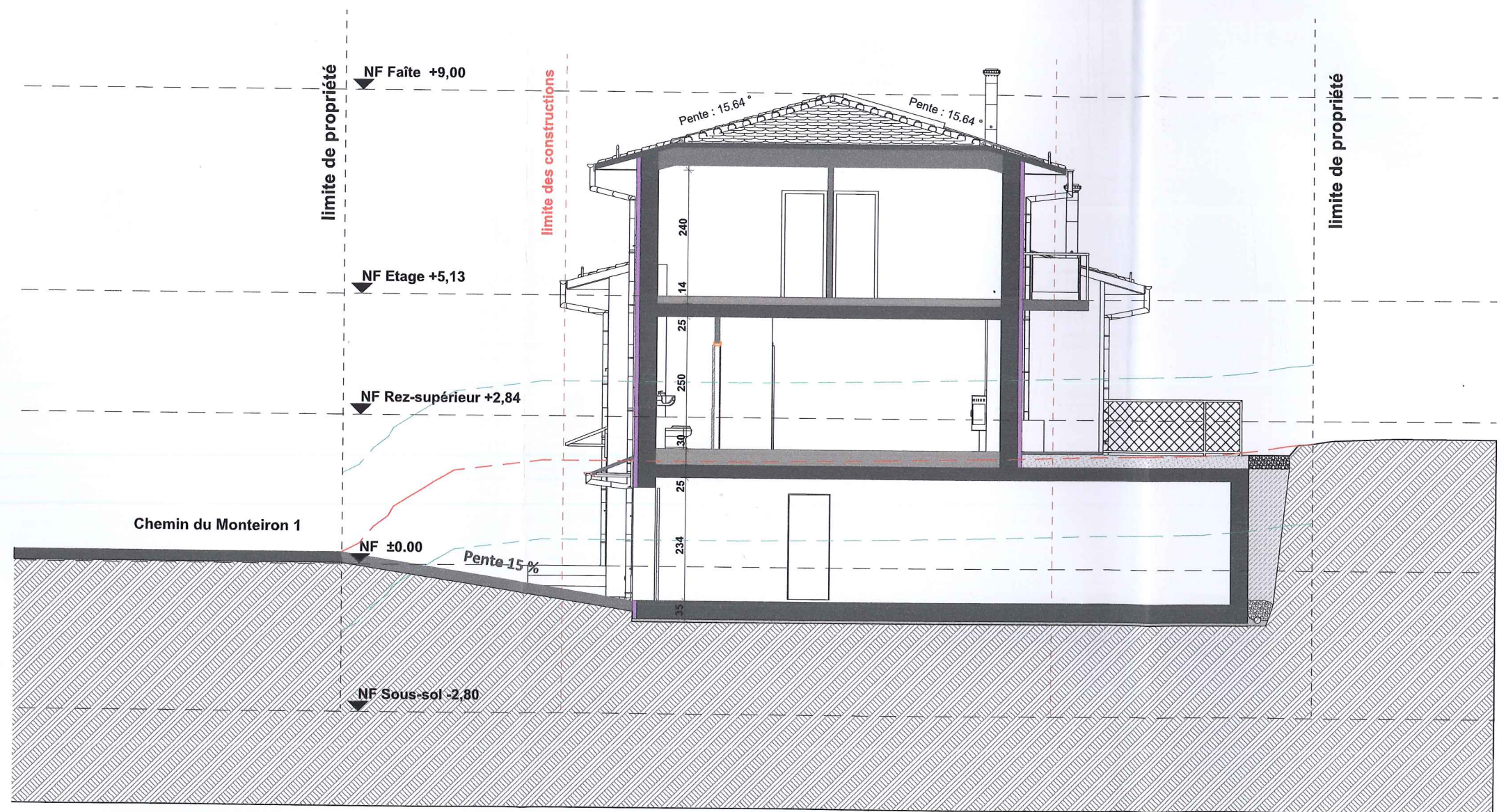
Coupe B1 1:100
