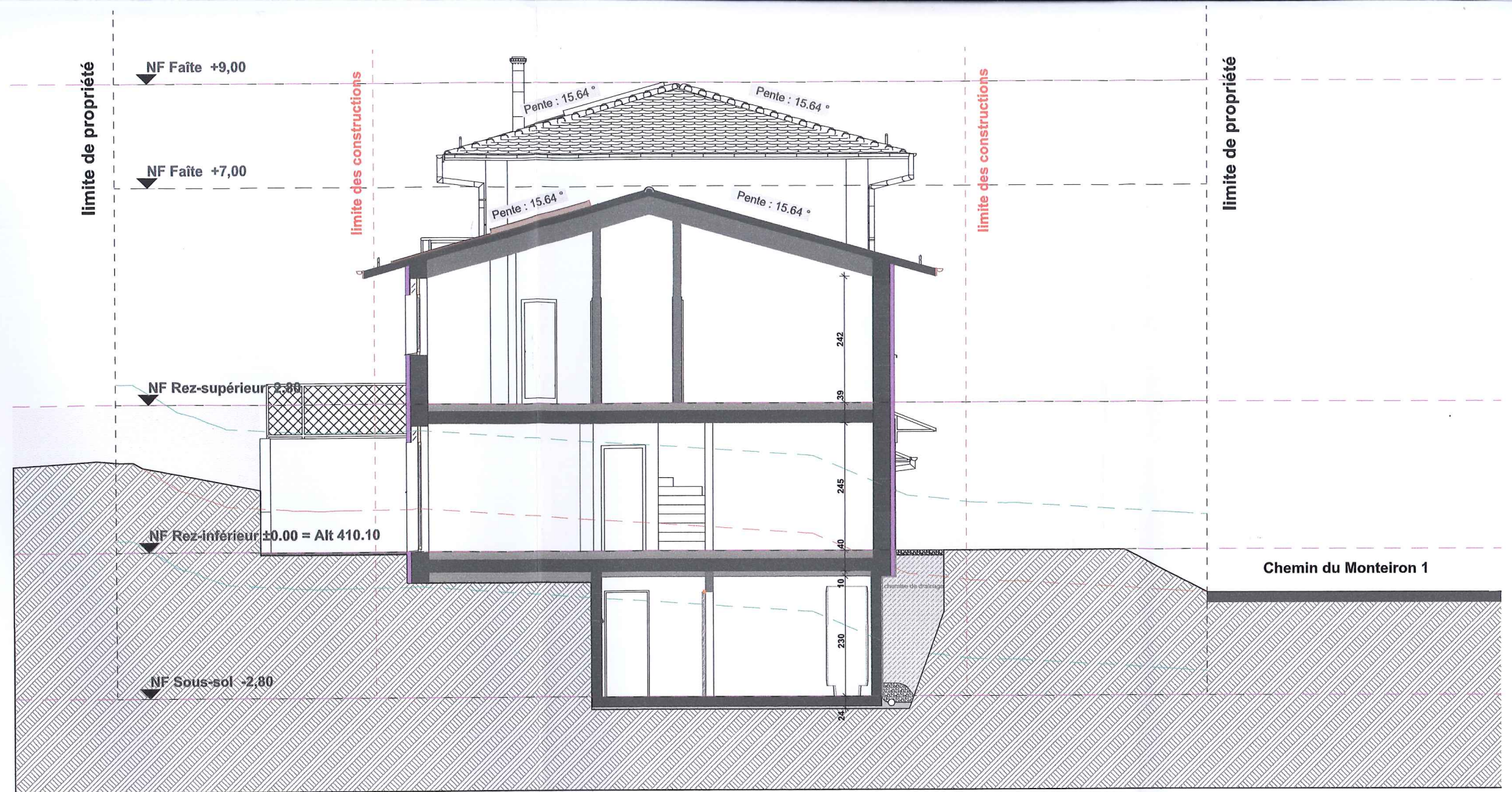
Coupe B3 1:100
