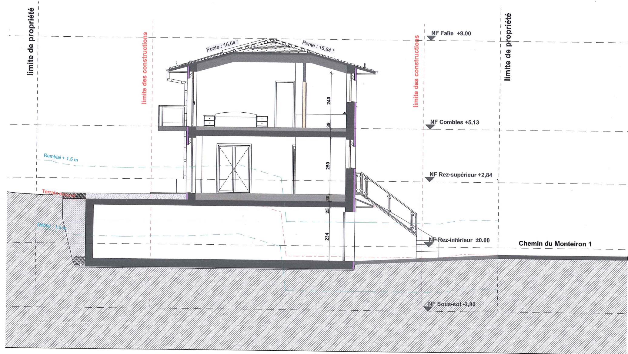
Coupe B2 1:100
