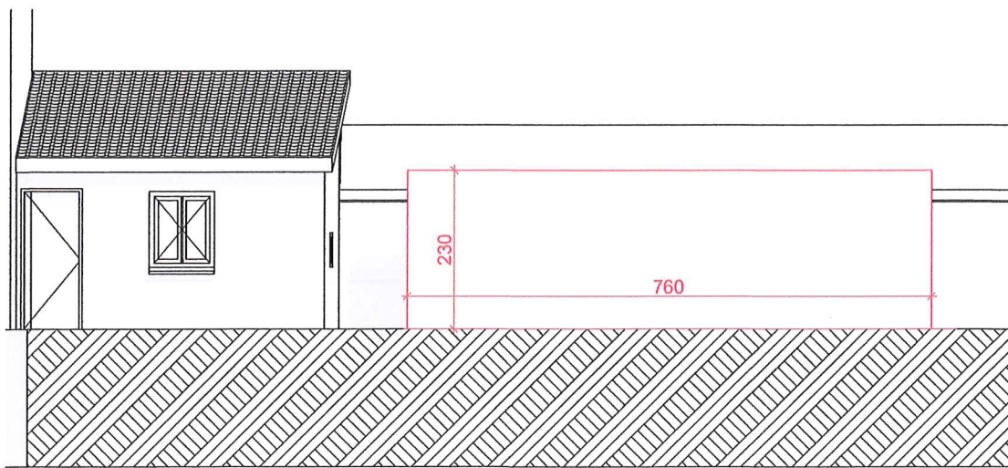
façade ouest
