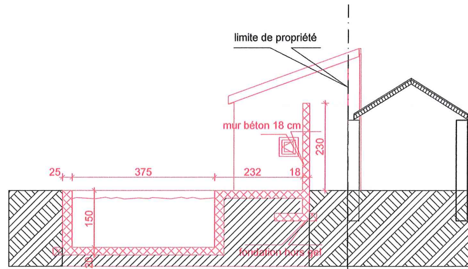
coupe AA
