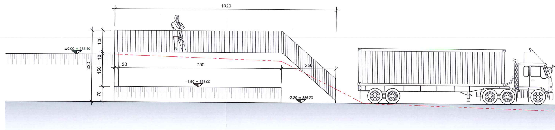
Elévation
